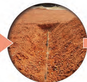
排水管を併称した水はけ対策
